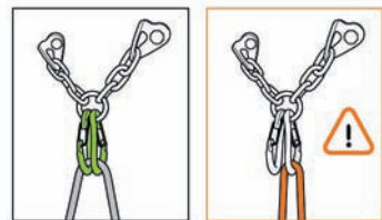
Inštalácia lana do kotviaceho bodu
